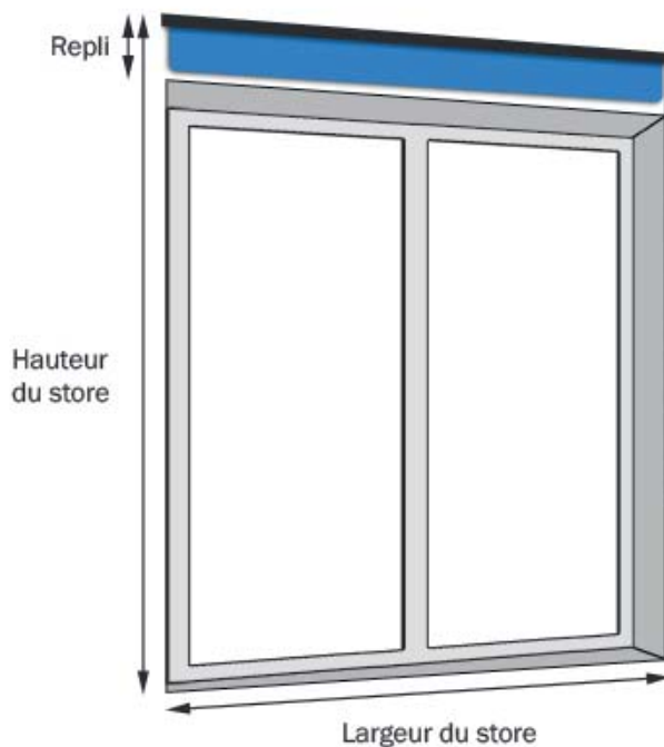
POSE EN FAÇADE
